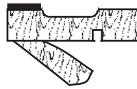
Kantenzwinge
